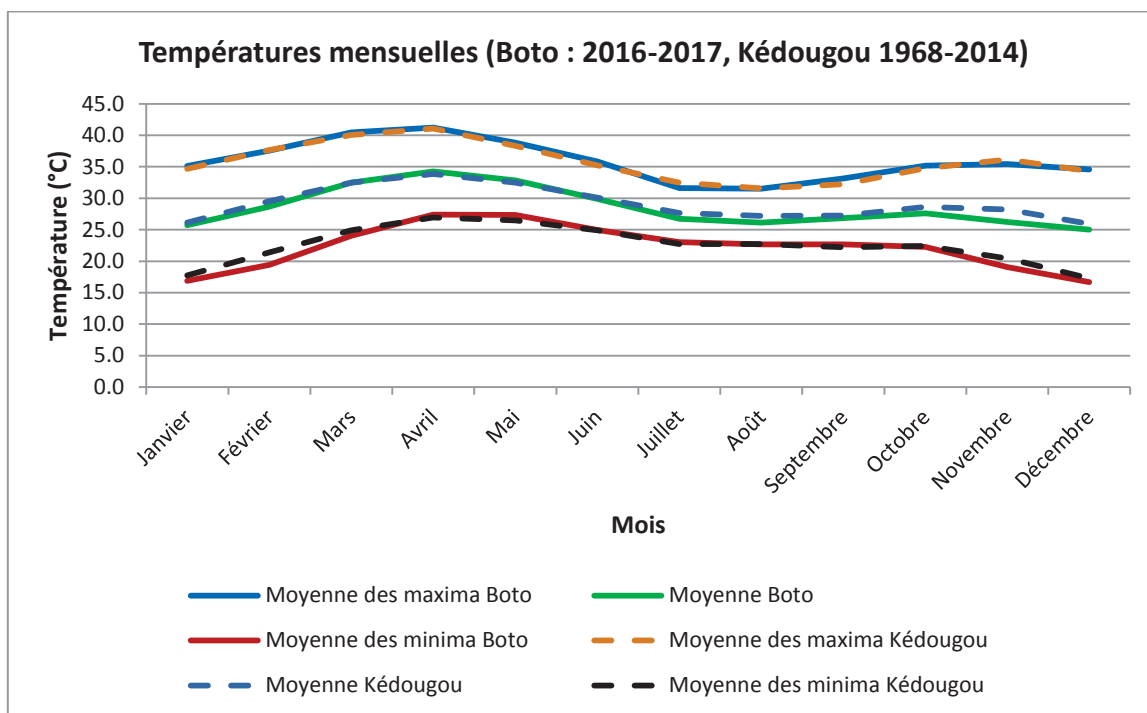
Figure 4.1.2 Régime thermique à la station météorologique de Kédougou (1968-2014) et comparaison avec les données de Boto (2016-2017)
