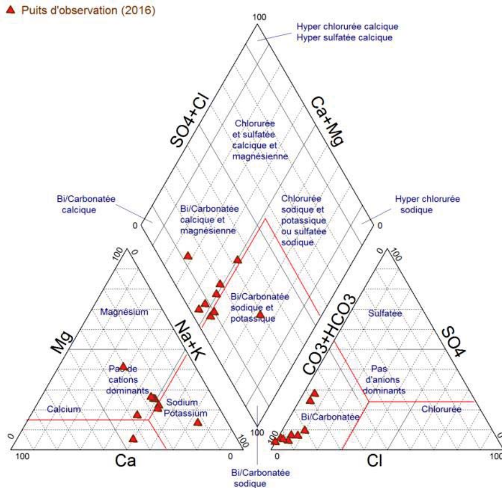
Figure 4.1.14 Diagramme de Piper des eaux des puits d'observation (2016)
